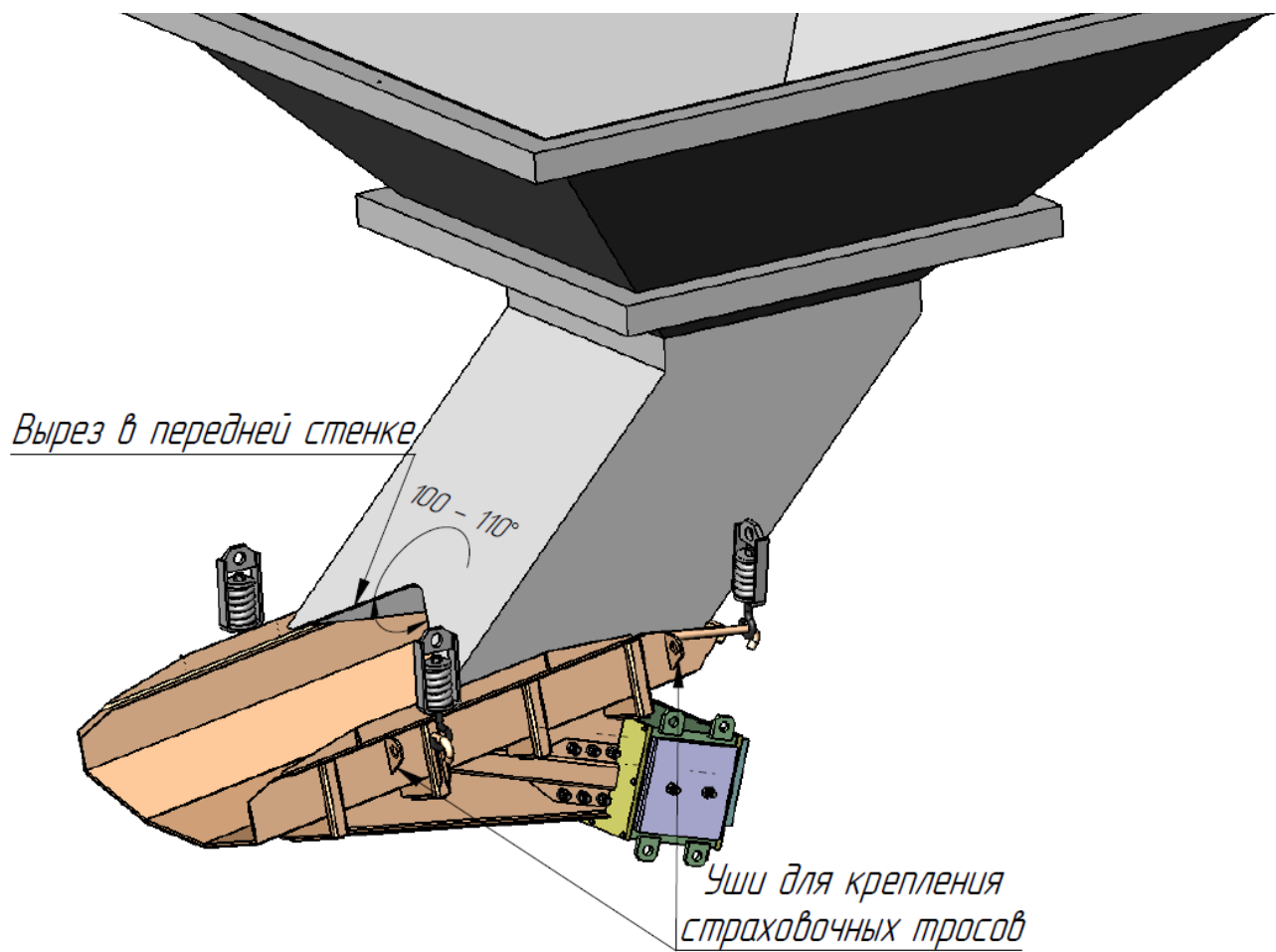
Рис.5 Установка питателя под бункером.
