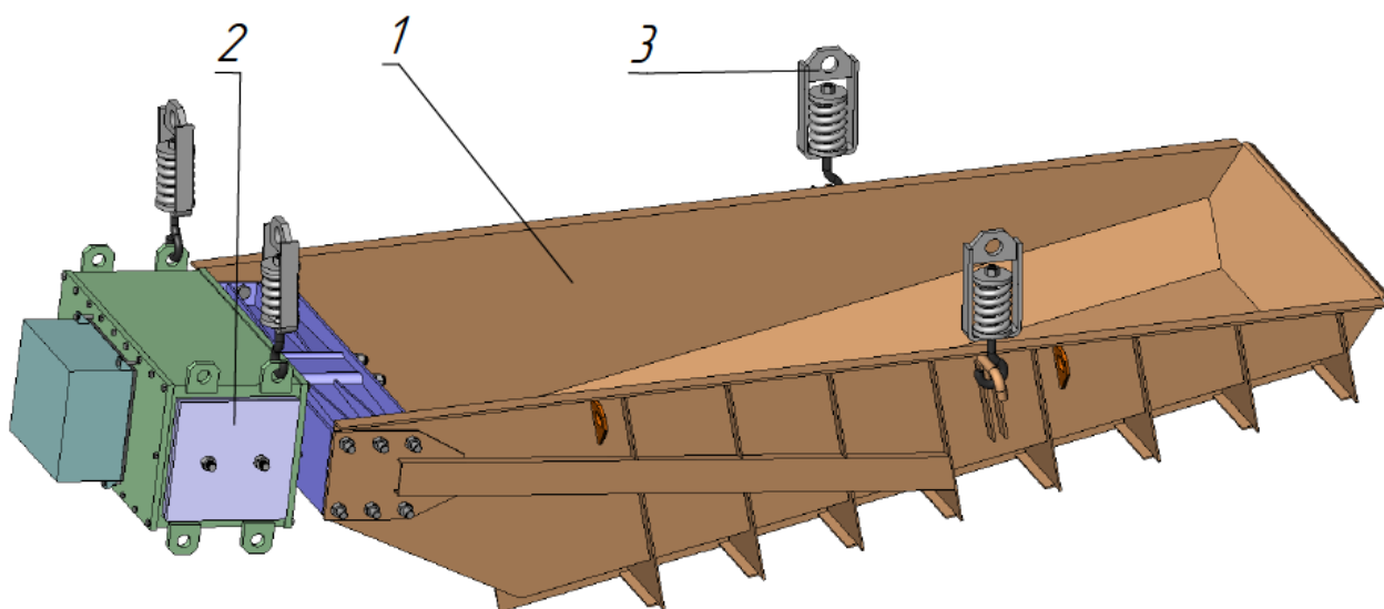
Рис.2 Вибропитатель с верхним расположением привода.
