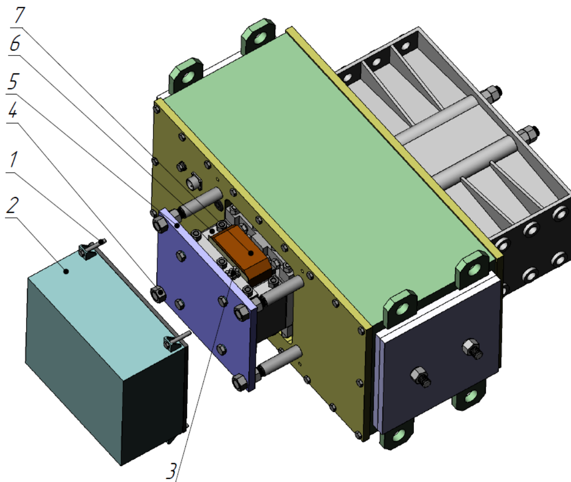
Рис.8-1 Замена катушки электромагнита
