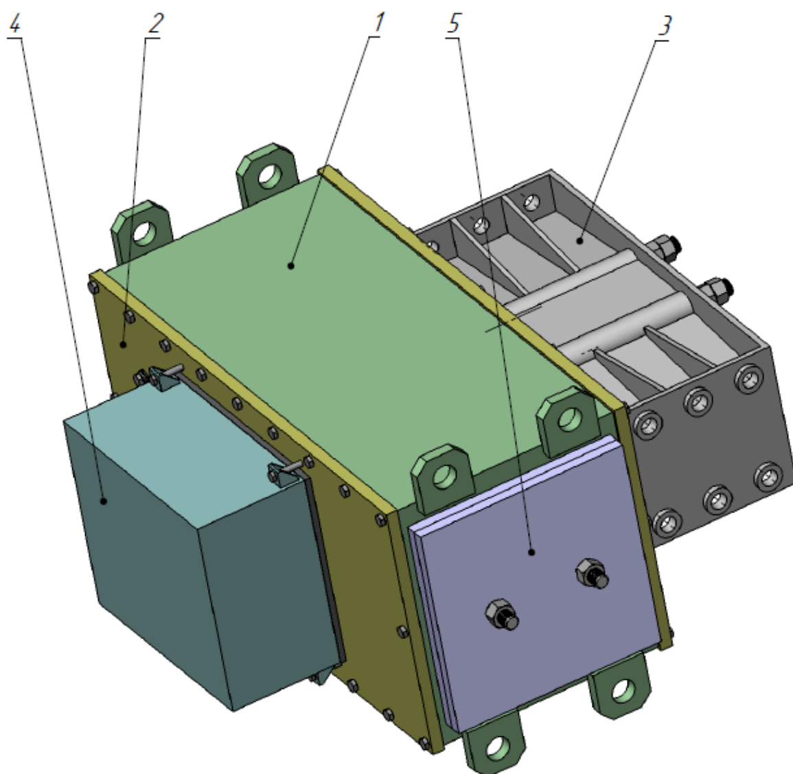
Рис.3 Вибропривод рессорный одноконтный.
