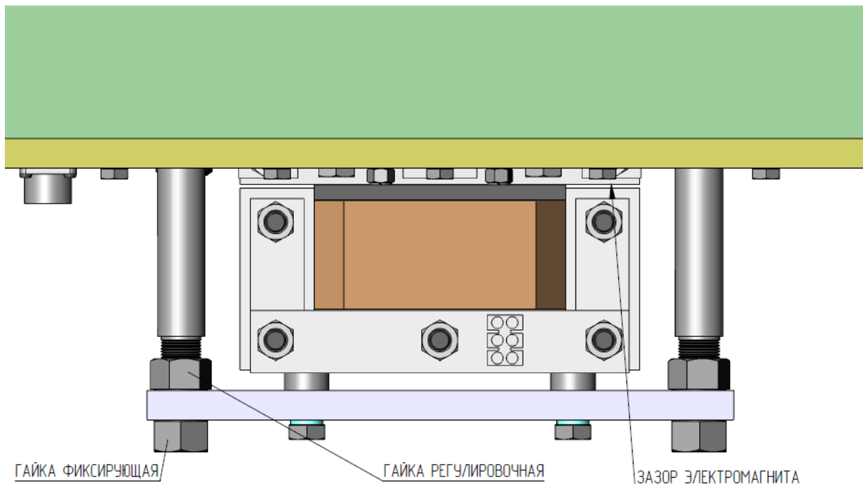
Рис.7 Регулировка зазора электромагнита
