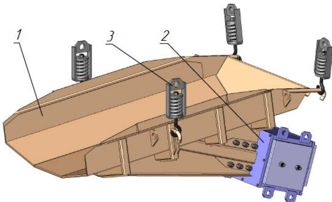
Рис.1 Вибропитатель с нижним расположением привода.
