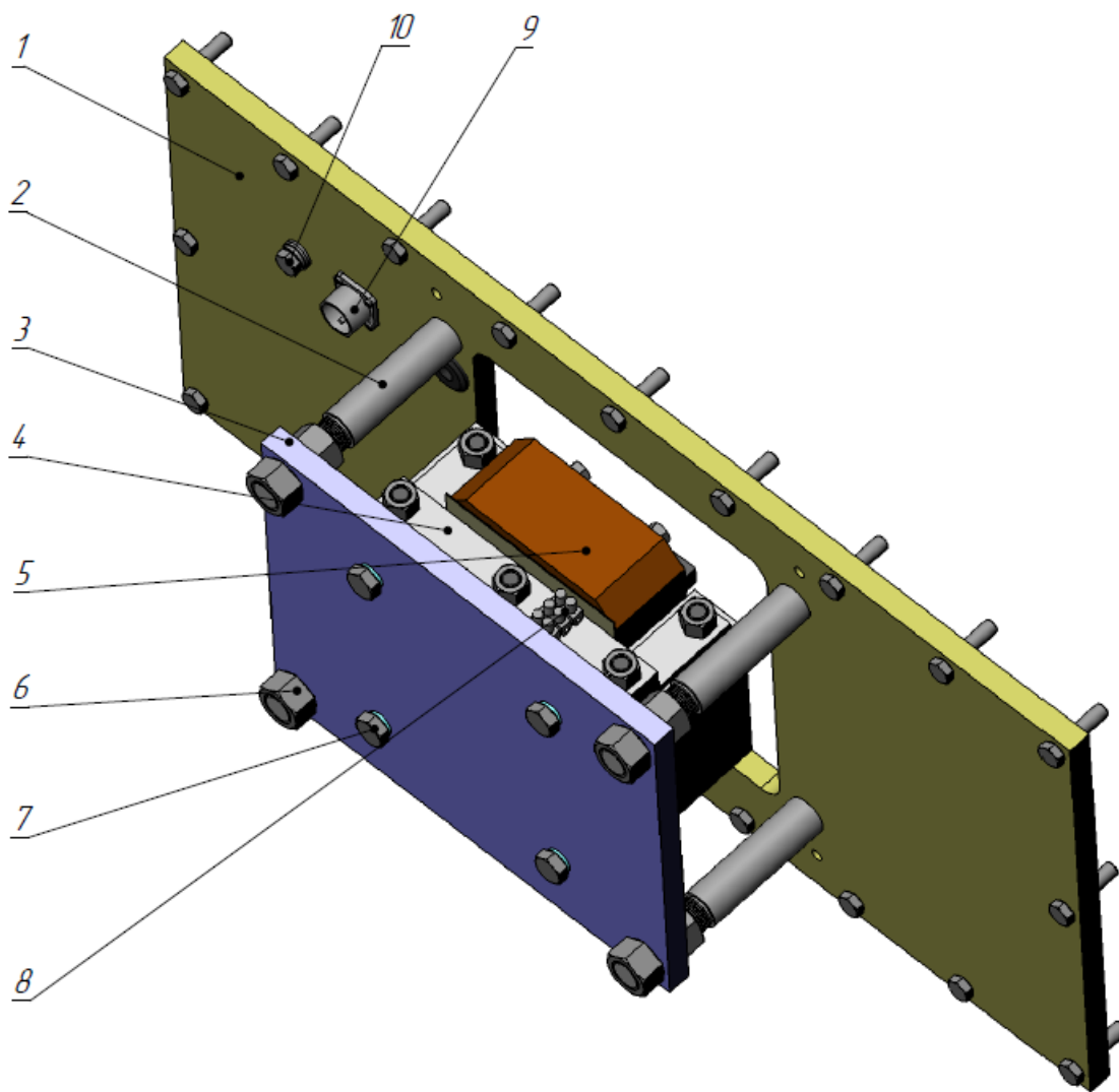
Рис.4 Крышка задняя в сборе. Кожух условно не показан.
