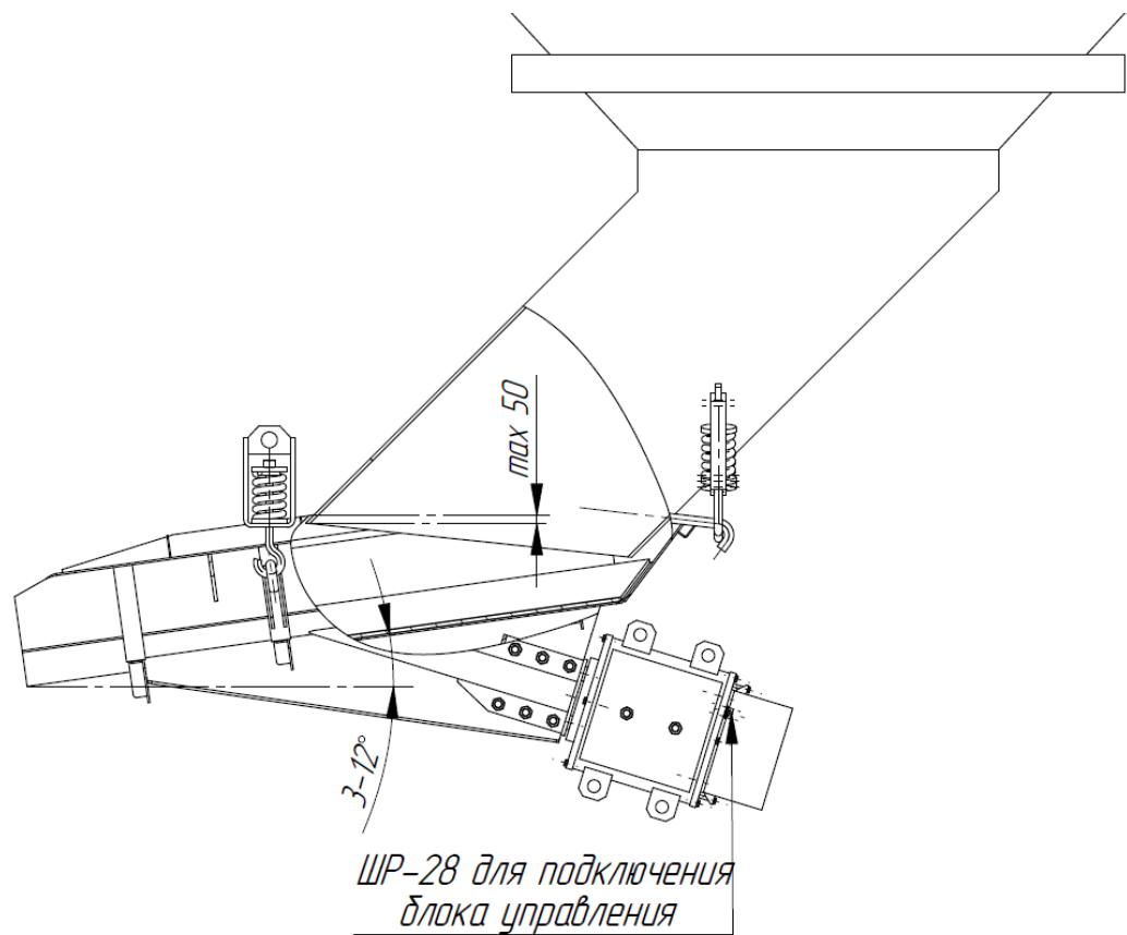
Рис .6 Установка питателя под бункером. Вид сбоку.
