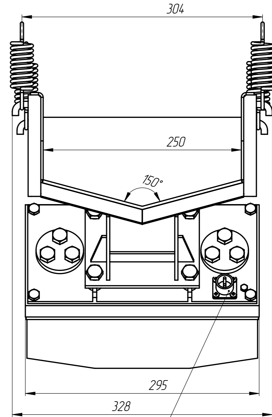
ШР-20 для подключения блока управления
