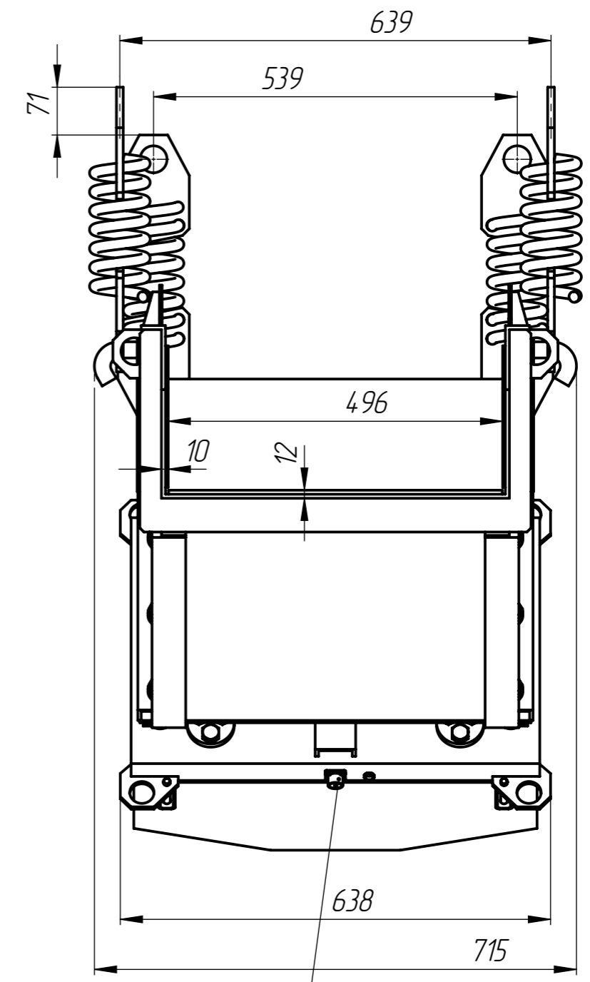
ШР-20 для подключения блока управления
