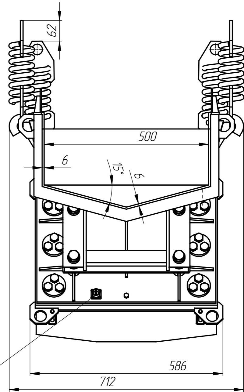
Разъем ШР-20 для подключения блока управления
