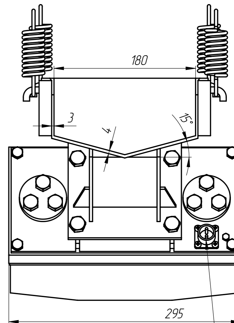
Разъем ШР-20 для подключения блока управления
